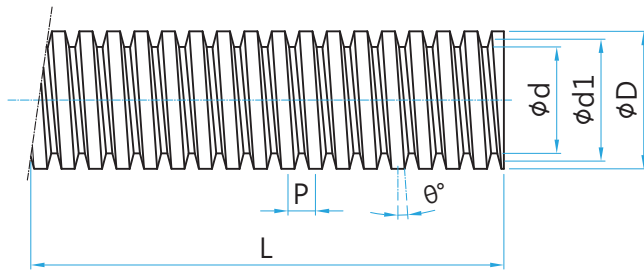
TMSR 오른나사형상
